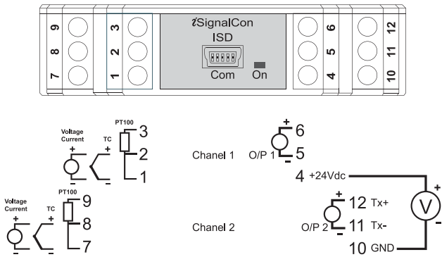
圖2. 配線端子說明
